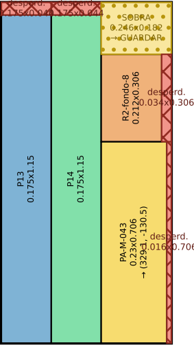
Pieza M-26 · 4 recorte(s)
