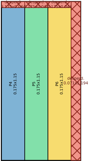
Pieza M-91 · 3 recorte(s)
