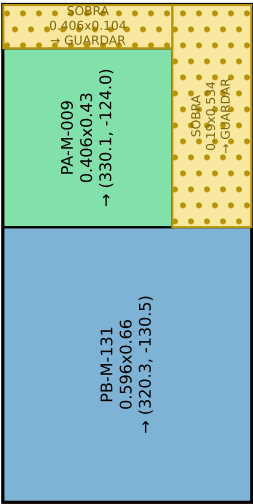
Pieza M-13 · 2 recorte(s)
