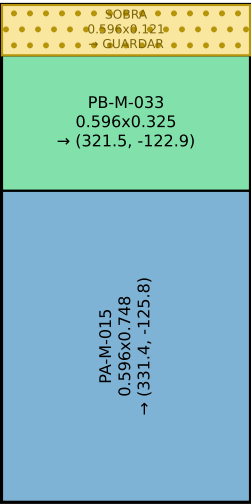
Pieza M-14 · 3 recorte(s)
