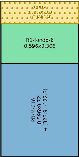
Pieza M-36 · 2 recorte(s)
