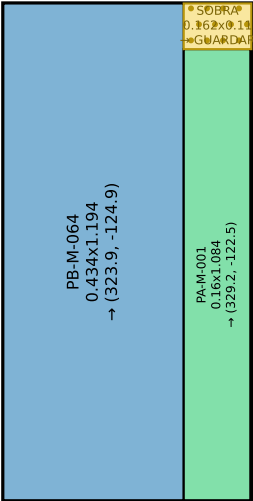
Pieza M-16 · 2 recorte(s)
