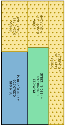
Pieza M-08 · 2 recorte(s)
