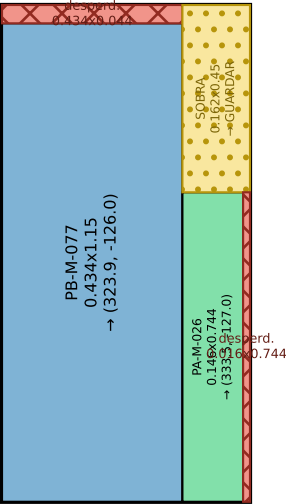
Pieza M-32 · 1 recorte(s)
