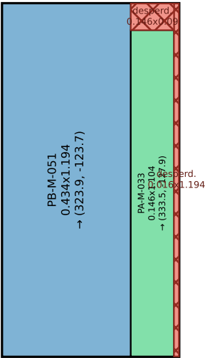
Pieza M-33 · 1 recorte(s)
