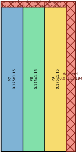
Pieza M-92 · 3 recorte(s)
