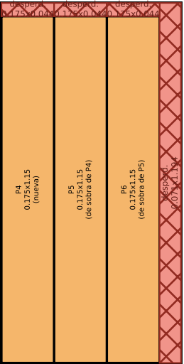
Pieza M-91 (misma del plan general)
